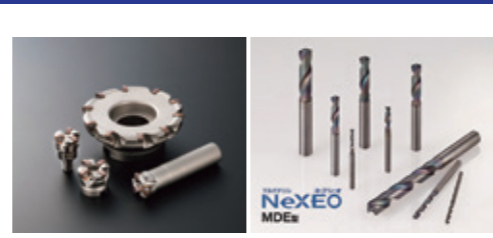
SEC-スミデュアルミル DMSW型
